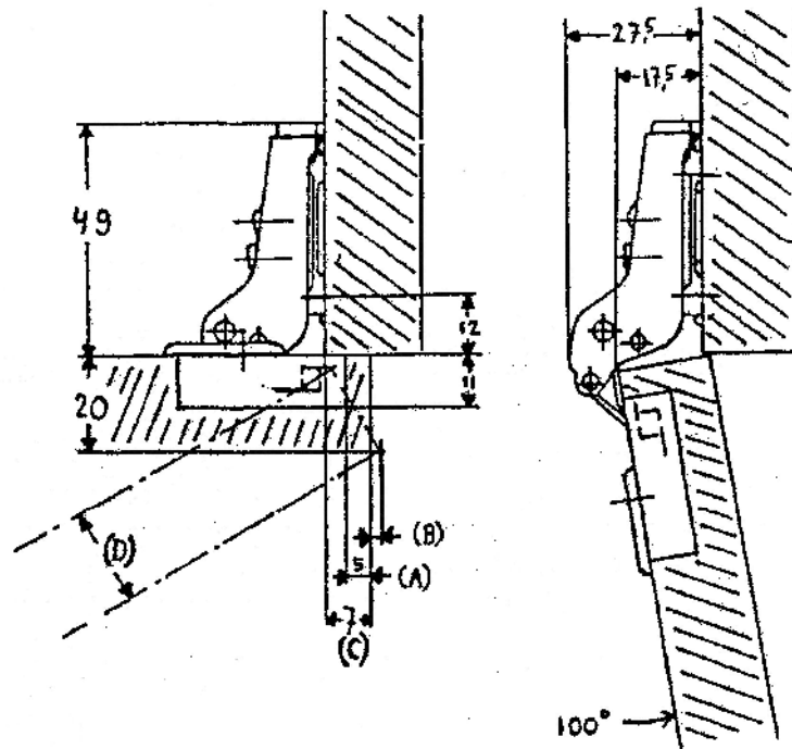
Mittelband 1274 VA
