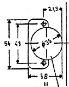
Bohrbild
