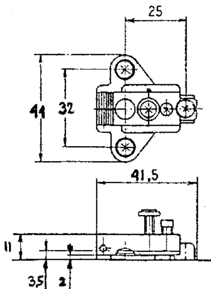
Grundplatte 1278VA
