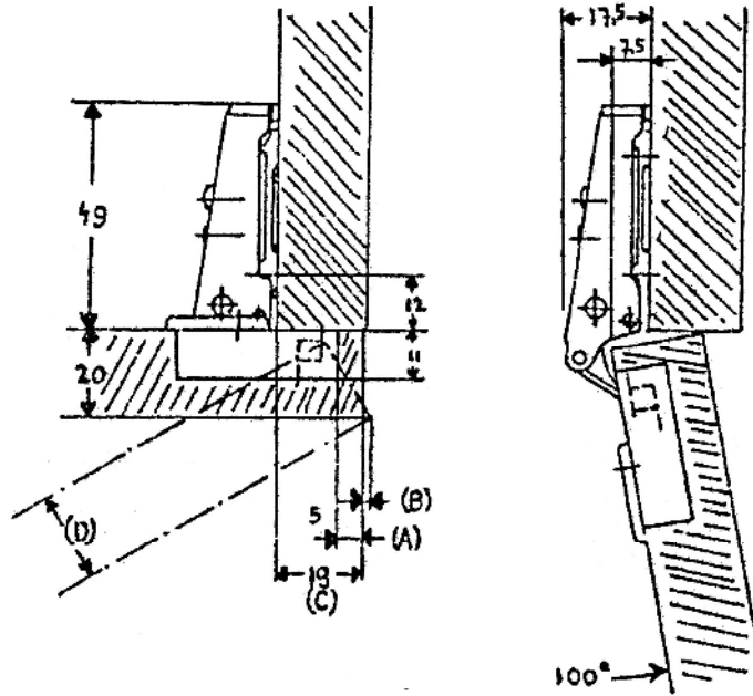
Eckband 1270 VA
